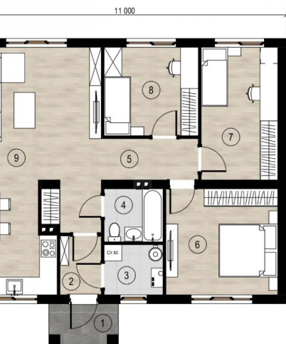
Планировочное решение 1-го этажа
