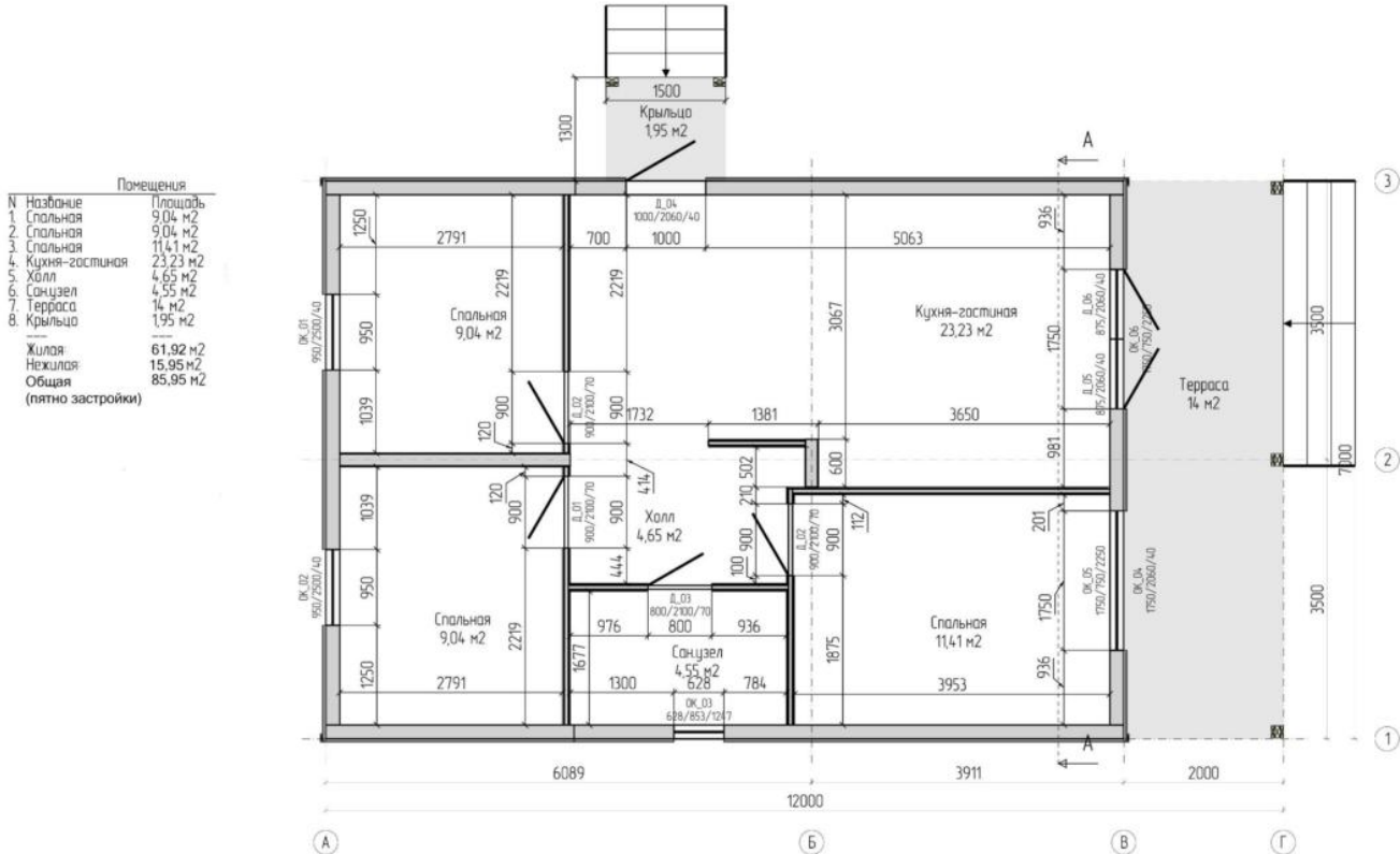
План дома:
