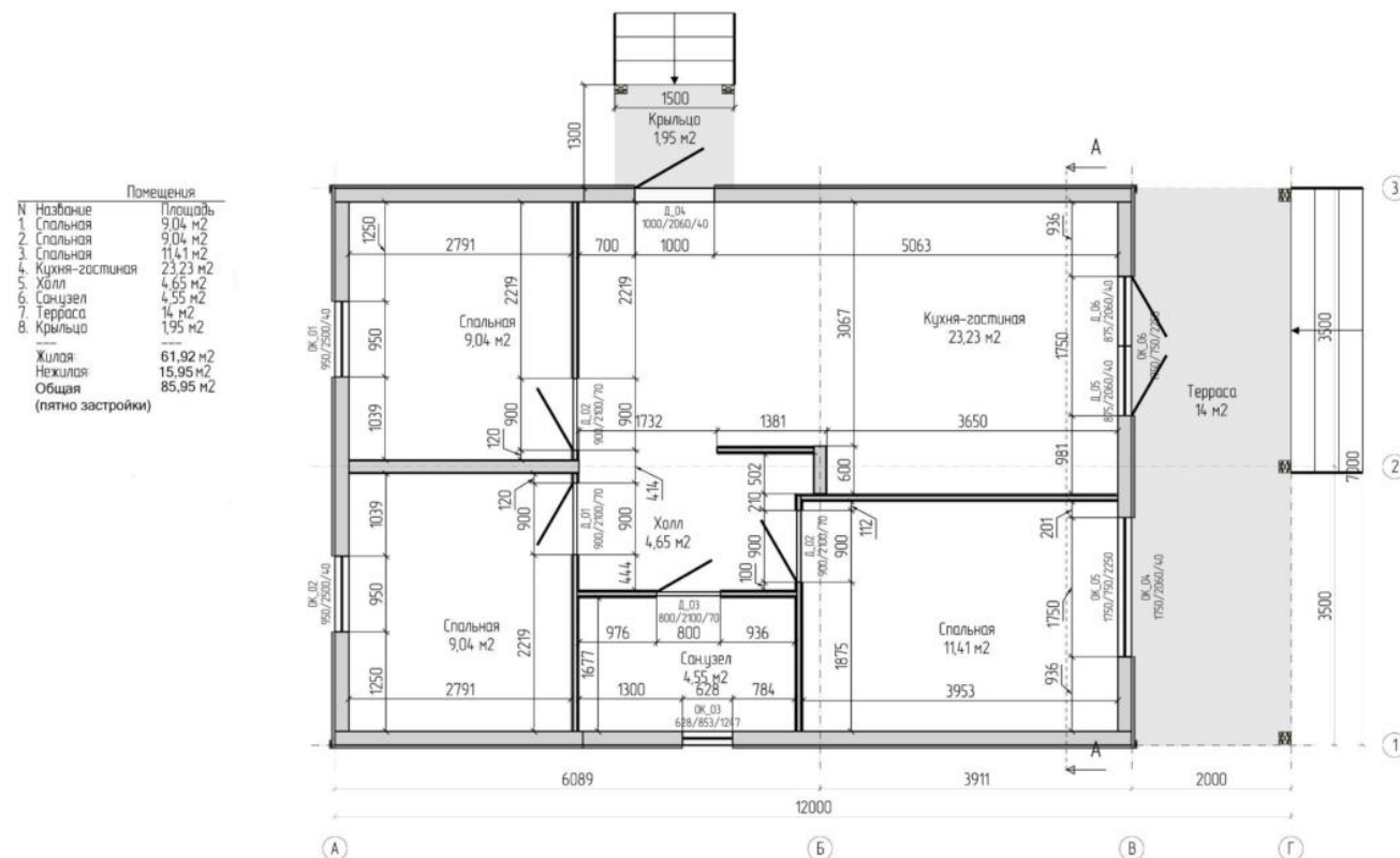
План дома:
